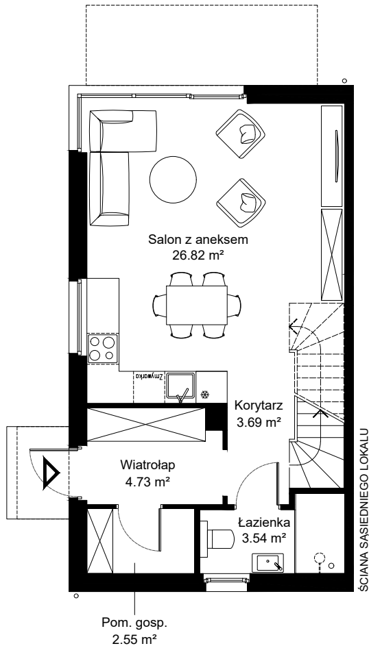
RZUT PARTERU
