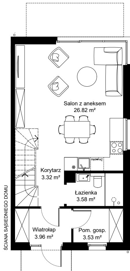
RZUT PARTERU
